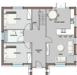
1.02 1F PLAN
